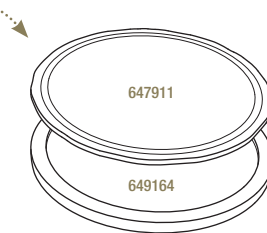
PLATEAU ROND POUR ASSIETTE À STEAK TRAY FOR ROUND STEAK PLATE
